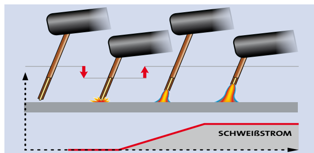
Höchst stabiler Lichtbogen und geringe Spritzerbildung. Durch die DIGITALE resonante Intelligenz wird eine noch schnellere Regelung als beim bewährten Resonanzinverter möglich.
